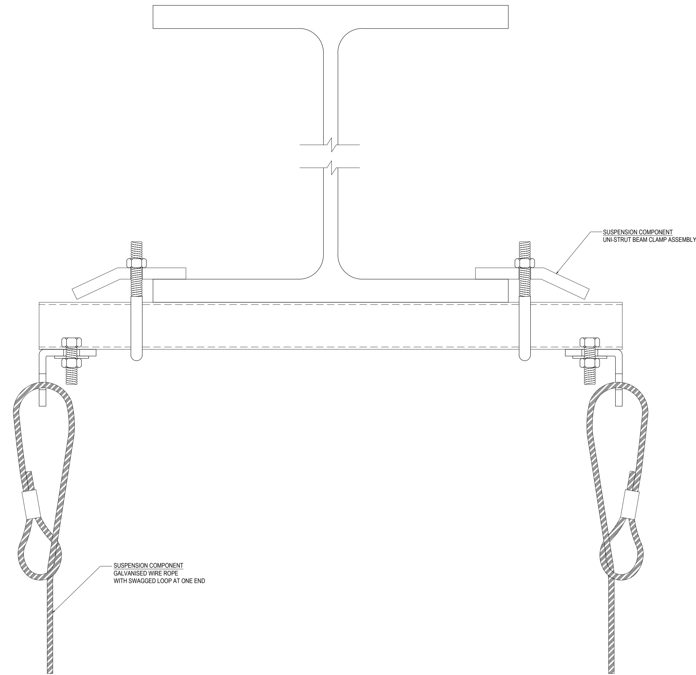
IWC-XCS-ML-18 SCALE 1:2
