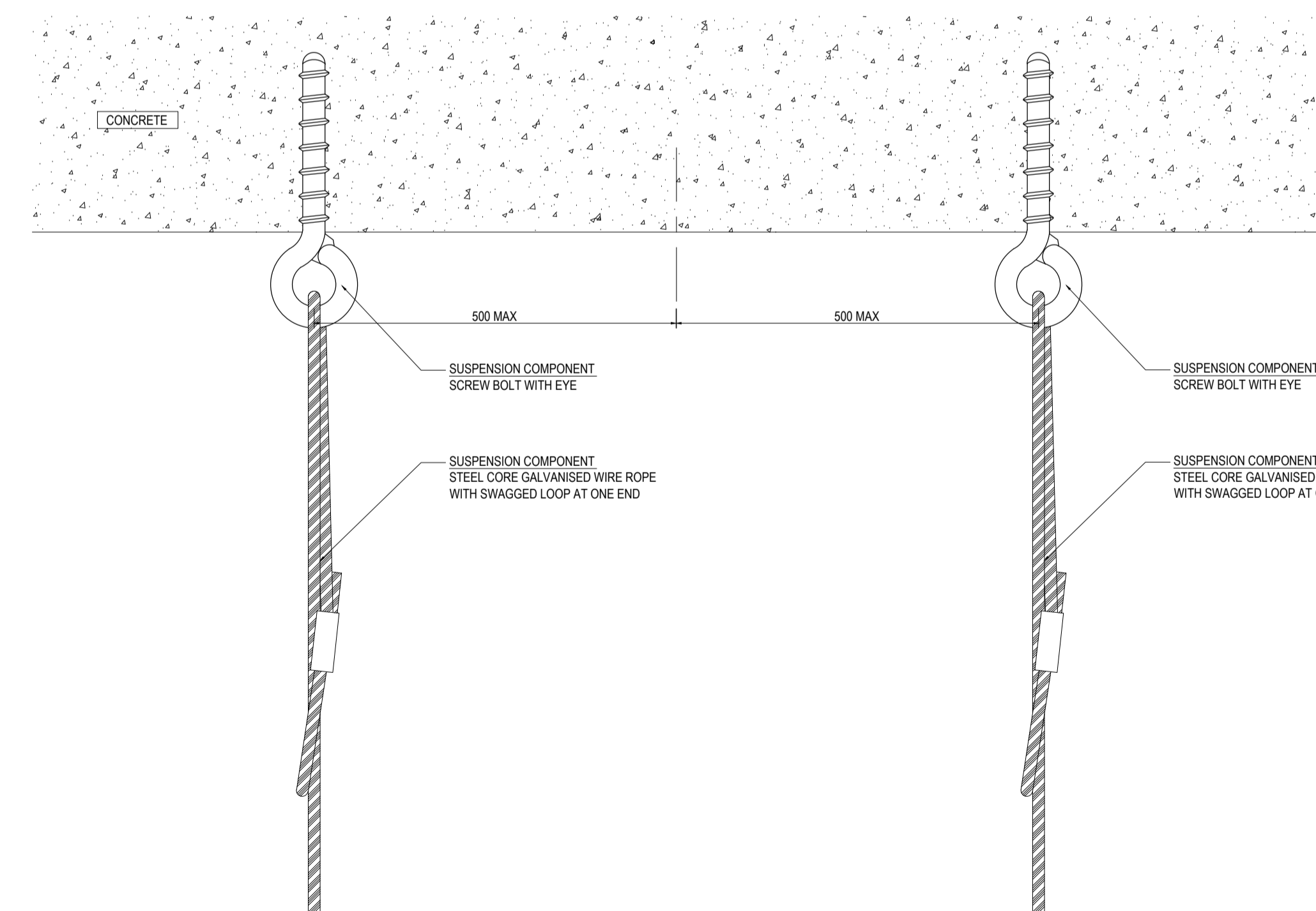
IWC-XCS-AT-14 SCALE 1:2
