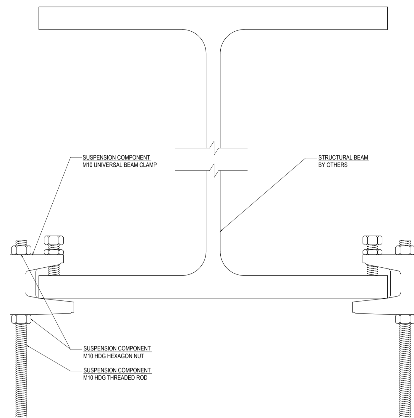
IWC-XCS-AT-17 SCALE 1:2
