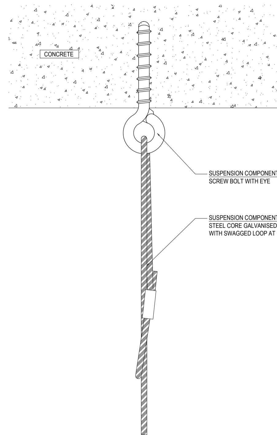
IWC-XCS-AT-07 SCALE 1:2
