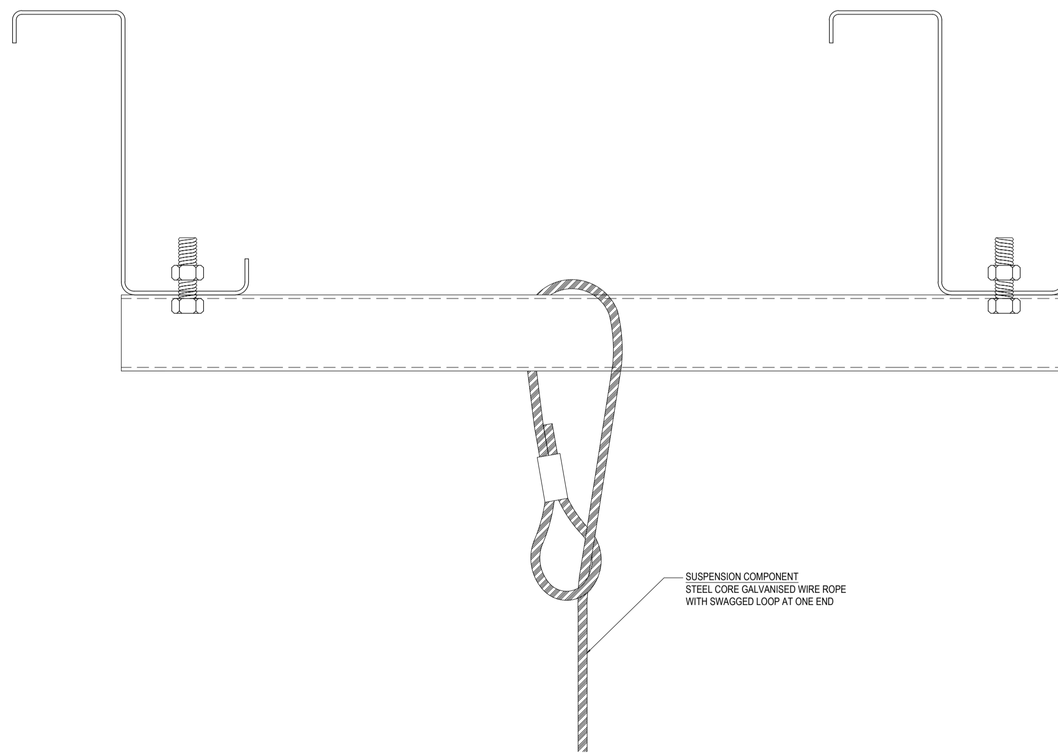
IWC-XCS-ML-19 SCALE 1:2
